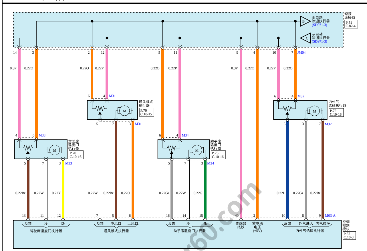
空调控制系统(自动)(2)
